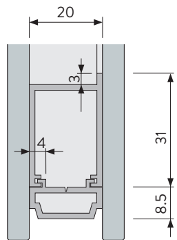
SECTION D-D
